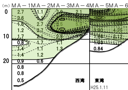
舞鶴湾 2013年(平成25年)1月 蛍光量
