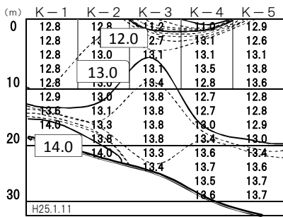
栗田湾 2013年(平成25年)1月 塩分濃度
