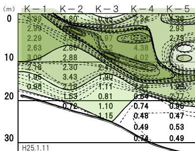
栗田湾 2013年(平成25年)1月 蛍光量
