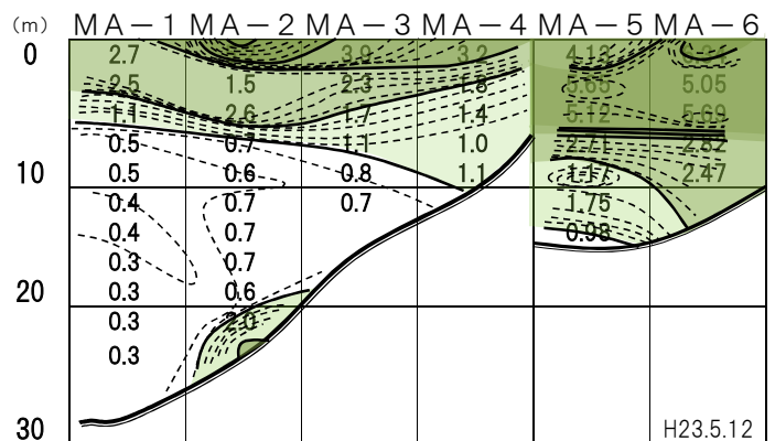
舞鶴湾 2011年(平成23年)5月 蛍光量
